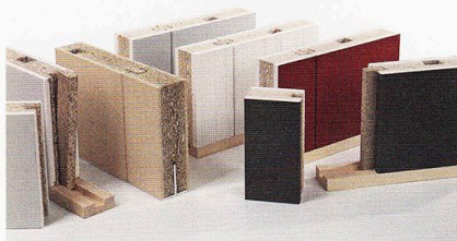
Sandwichbauweise mit dazwischenliegender Steinwolle.
